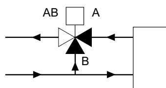
Bild 2 3-Wege-Ventil
