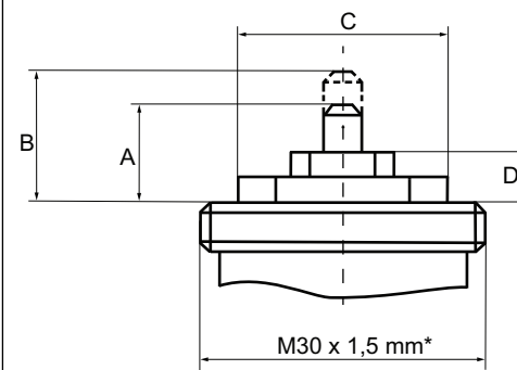
Figur 1 A = min. 9,0 mm; B = max 17,5 mm; C = max \varnothing 20,5 mm; D = max 9,0 mm, * Adaptorar med räckvidd M28 x 1,5 mm till M30 x 1,5 mm är tillgängliga. Kontakta Regin för mer information.
