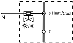
Bild 2 2-Rohr-Verdrahtung
