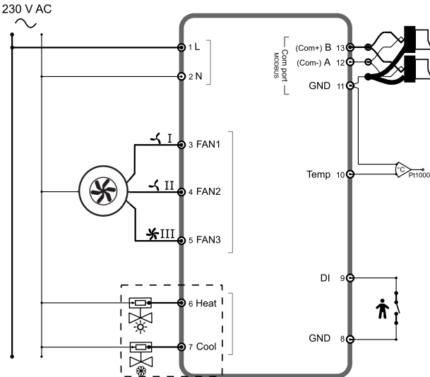
Bild 1 4-Rohr-Verdrahtung
