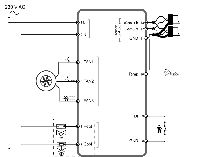
Fig. 1 Raccordement à 4 tubes
