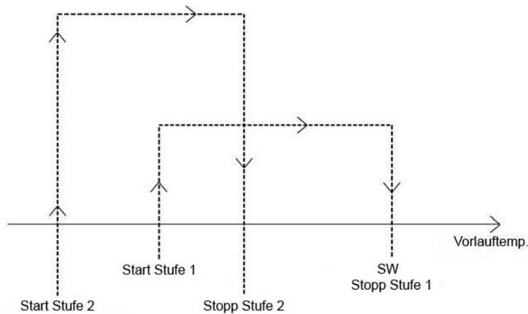
Bild 3-20 Aus/An-Regelung
