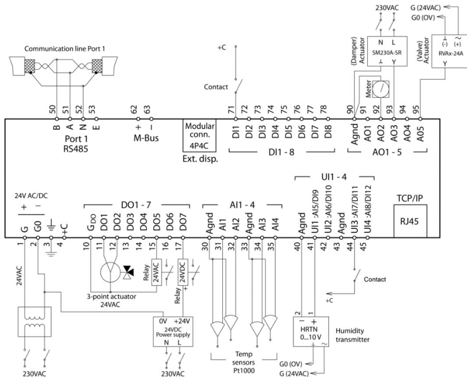
Bild 4-4 Klemmenbelegungsbeispiel
