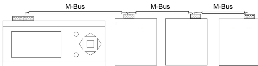
Bild 4-10 M-Bus Zähler
