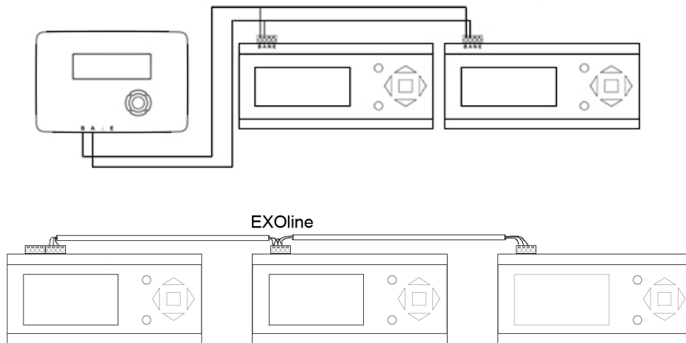
Bild 4-11 Erweiterungseinheiten über EXOline
