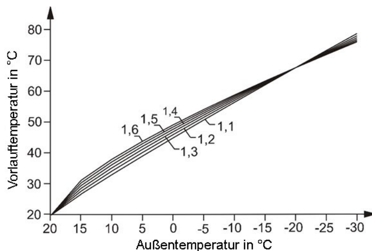
Bild 3-6 Exponent DIN-Kurve
