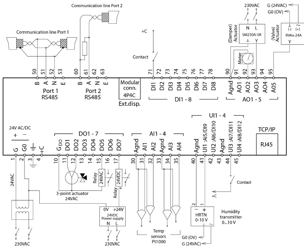
Bild 4-3 Klemmenbelegungsbeispiel
