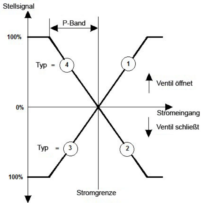
Bild 3-7 Universalbegrenzung
