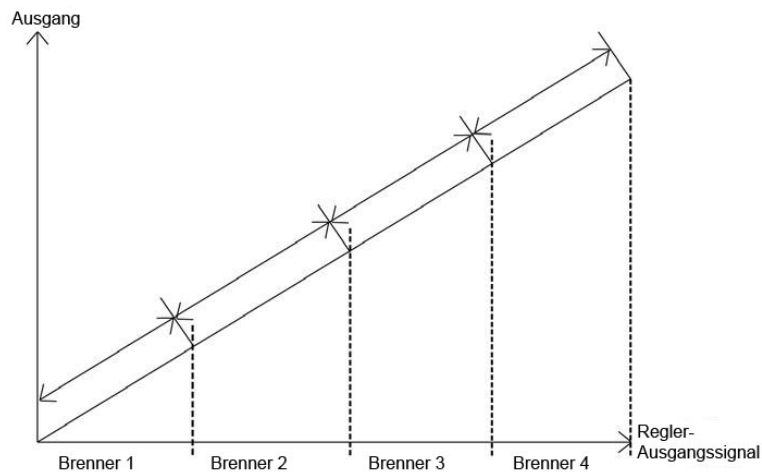
Bild 3-23 Regelung modulierend
