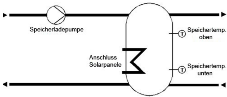
Bild 3-16 Pufferspeicher
