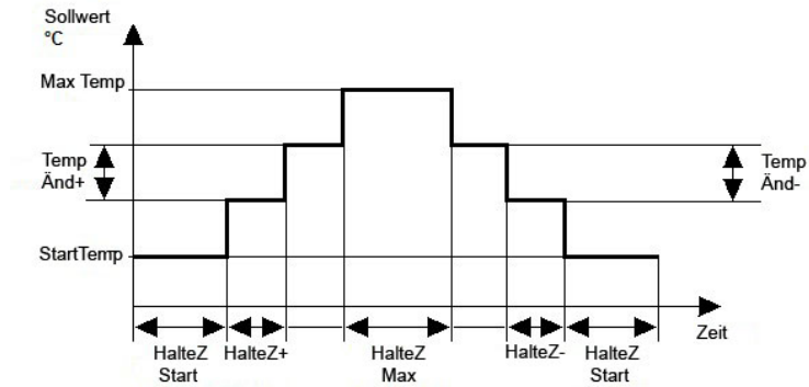
Bild 3-9 Estrichrocknung
