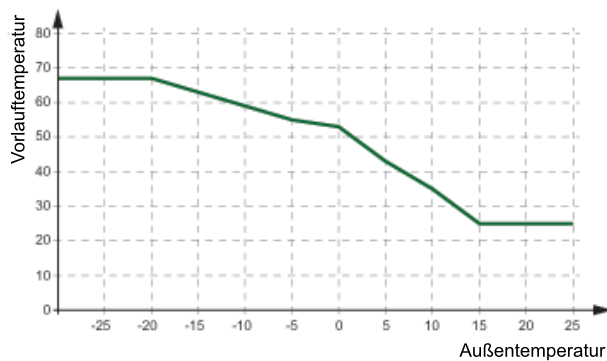
Bild 2-3 8-Punkt-Kennlinie
