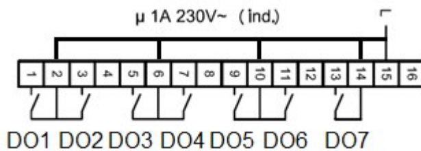
Bild 4-9 Digitalausgänge
