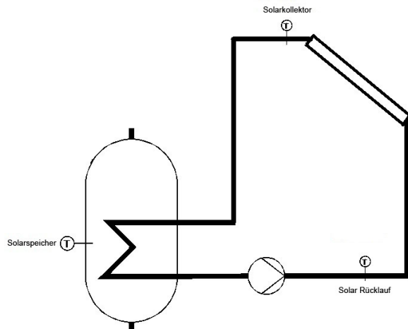
Bild 3-19 Solarkreis
