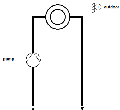
Bild 3-2 Ungemischter Heizkreis
