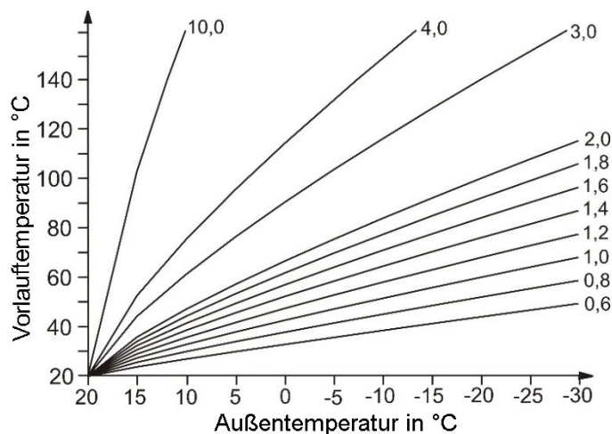
Bild 3-5 Steigung DIN-Kurve
