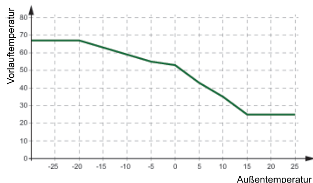
Bild 3-3 8-Punkt-Kennlinie
