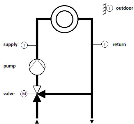
Bild 3-1 Gemischter Heizkreis
